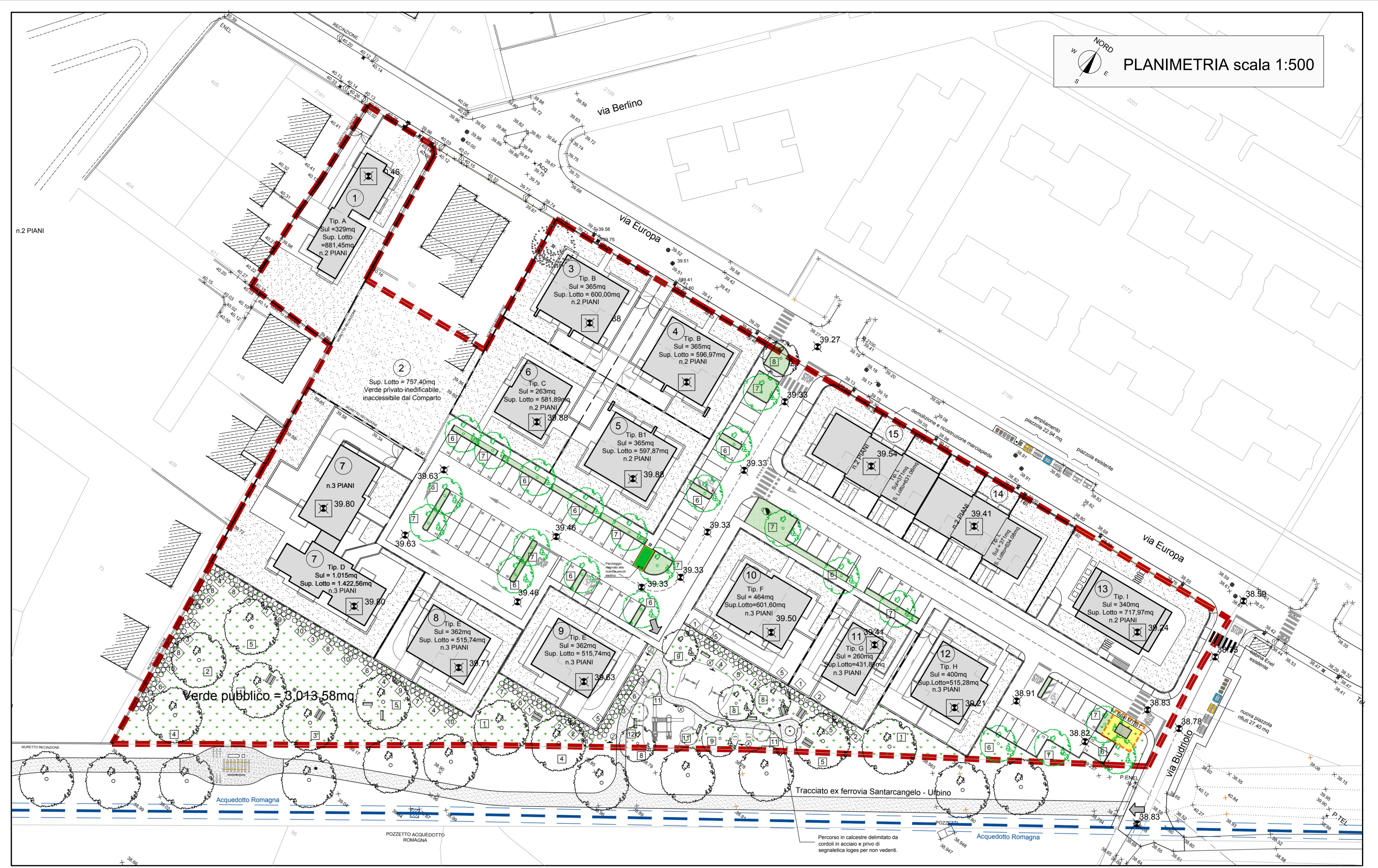
PLANIMETRIA scala 1:500
